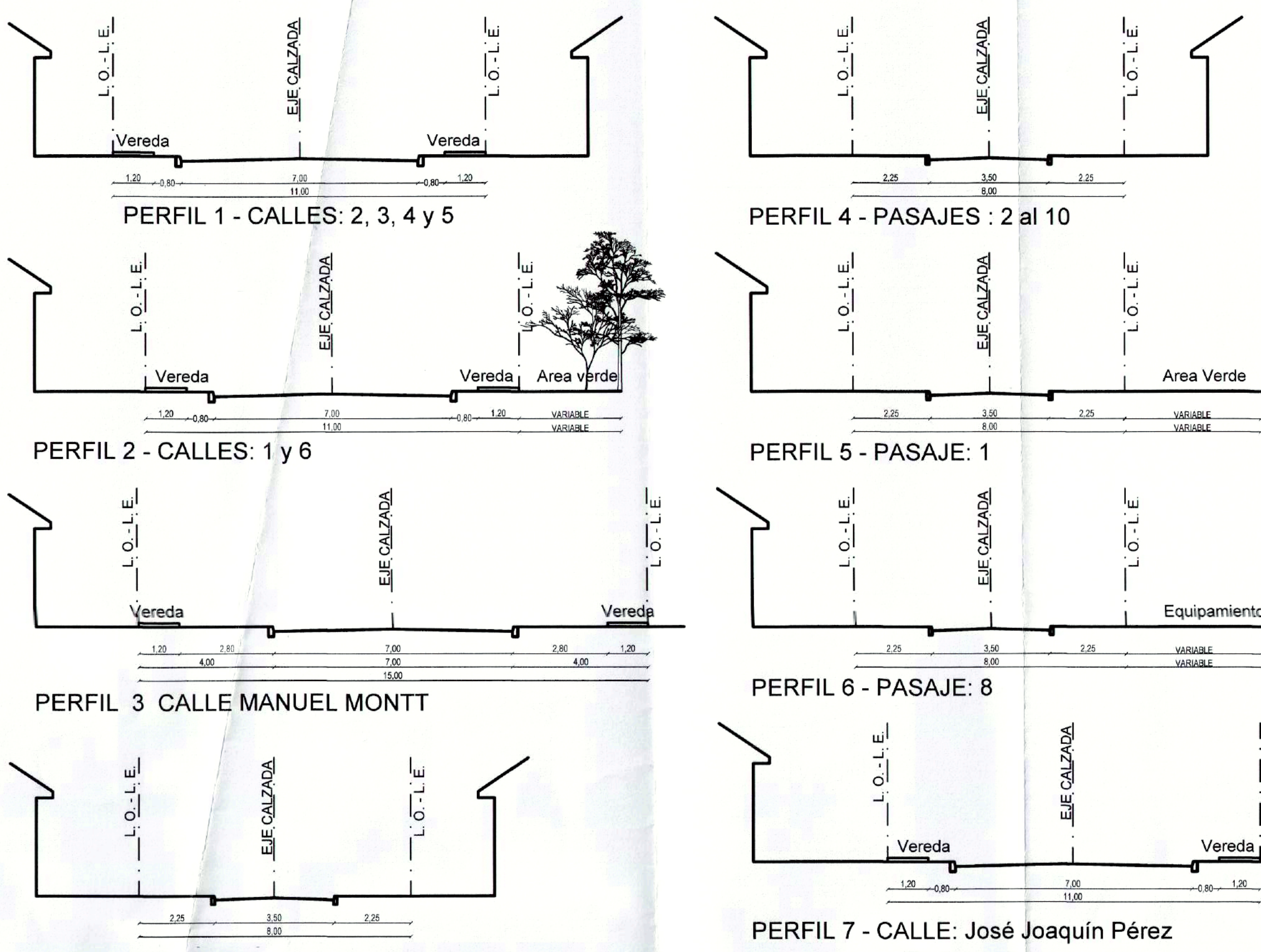
PERFILES PROYECTADOS escala 1/125
