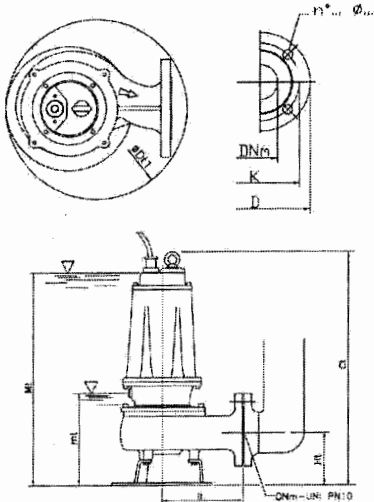
MOBILE INSTALLATION ПЕРЕДВИЖНАЯ ВЕРСИЯ DV 150-1000
