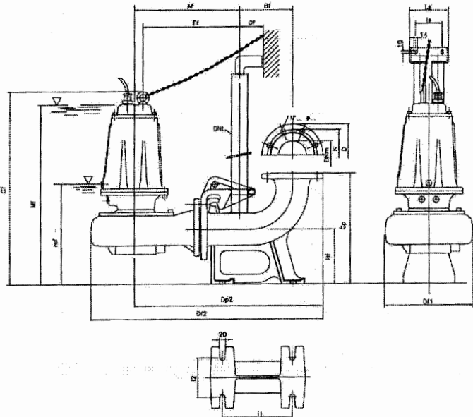
FIXED INSTALLATION WITH QUICK COUPLING KIT СТАЦИОНАРНАЯ ВЕРСИЯ С КОМПЛЕКТОМ ДЛЯ БЫСТРОЙ СБОРКИ DV 150-1000/P
